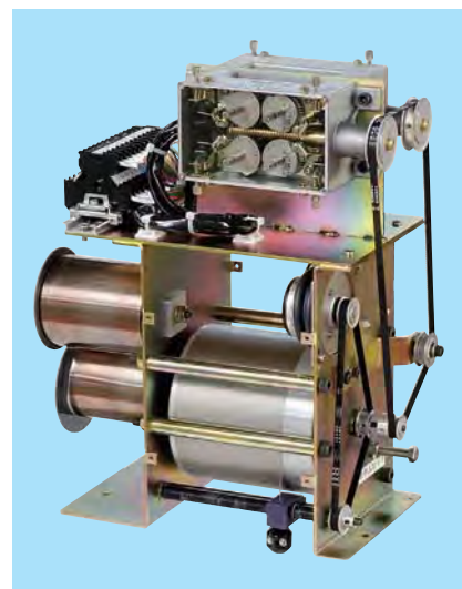
ワイヤリール (ストローク検出用)
