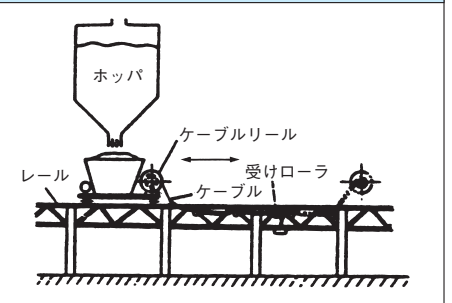
自走台車 ※
