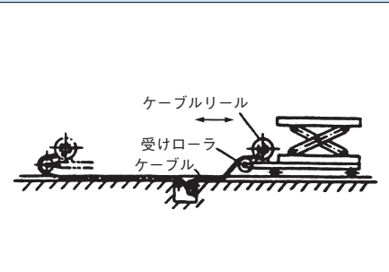
移動装置 ※
